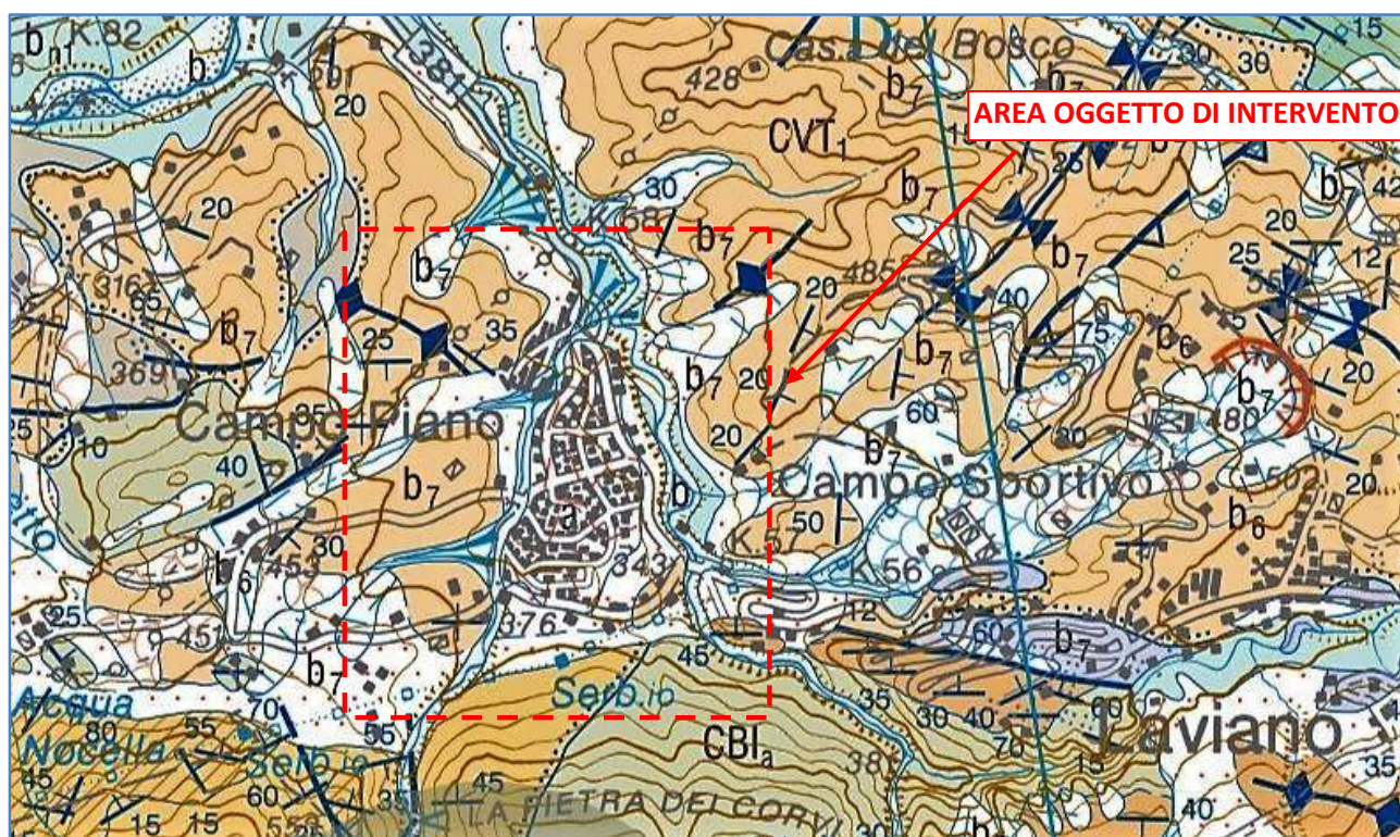
Fig. 3: Stralcio della Carta Geologica in scala 1:50.000 - F°468 Eboli. - Progetto CARG.
