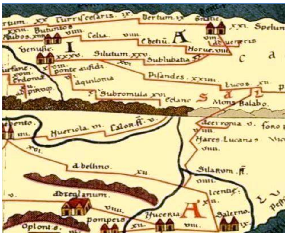
Fig. 5: la viabilità in Italia meridionale riportata nella Tabula Peutingeriana; a destra, l'indicazione del Mons Balabus , verosimilmente corrispondente al Monte Valva
